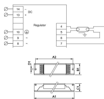
Specifikationer Philips HF-R 158 TL-D EII 220-240V for 1x58W
